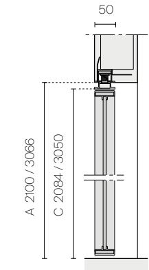
Wall flush swing door
