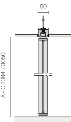
Ceiling flush swing door
