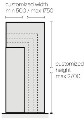
Door panel dimensions
