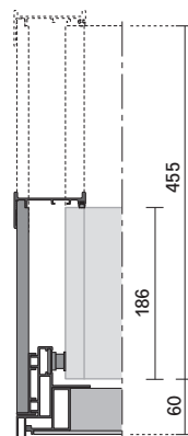
passaggio completo E45 complete passage E45 estensibile da mm 186 a mm 455 extensible from mm 186 to mm 455
