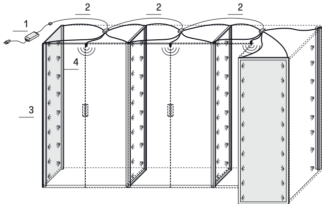
illuminazione anteriore e posteriore / front and back led lighting
