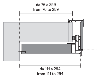
passaggio con fascia laterale su misura passage with customized lateral filler
