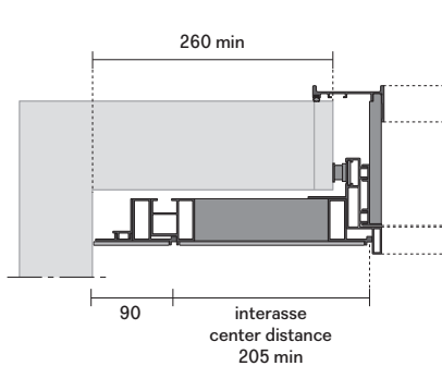
passaggio con pannello passage with panel
