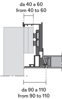
porta con fascia di aggiustaggio laterale door with adjustable lateral filler
