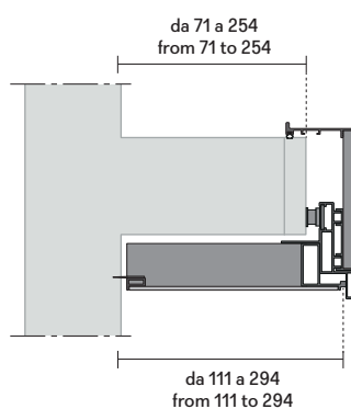
fascia terminale con fascia laterale su misura terminal closing filler with customized lateral filler
