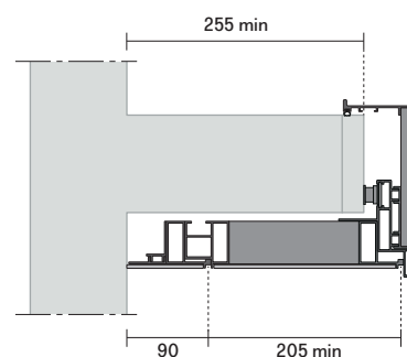
fascia terminale con fascia di aggiustaggio laterale e pannello / terminal closing filler with adjustable lateral filler and panel
