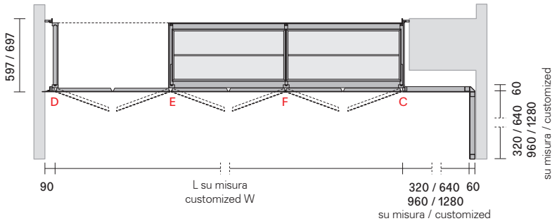
composizione interparete con contenitori e vano di passaggio laterale niche composition with storage units and side passage opening
