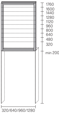
struttura sopra luce fanlight structure
