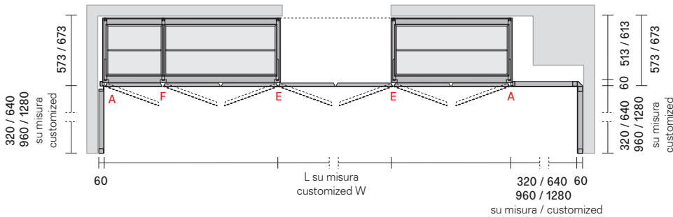
composizione articolata con contenitore angolare articulated composition with corner storage unit
