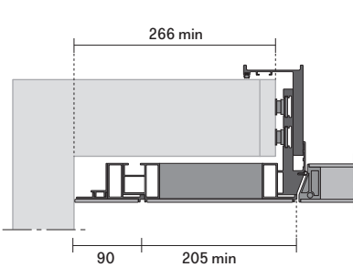
porta con fascia di aggiustaggio laterale e pannello door with adjustable lateral filler and panel
