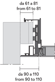
porta con fascia di aggiustaggio laterale door with adjustable lateral filler
