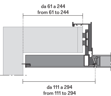
porta con fascia laterale su misura door with customized lateral filler
