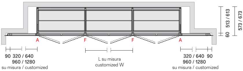
composizione lineare con contenitore centrale linear composition with central storage unit
