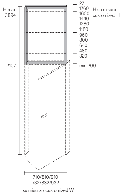
struttura sopraluce porta door fanlight structure
