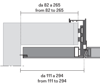
porta con fascia laterale su misura door with customized lateral filler
