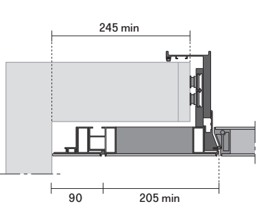
porta con fascia di aggiustaggio laterale e pannello door with adjustable lateral filler and panel
