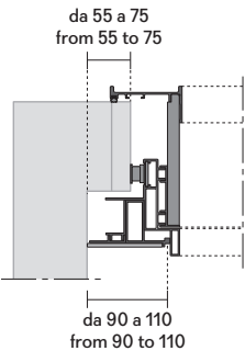
passaggio con fascia di aggiustaggio laterale passage with adjustable lateral filler
