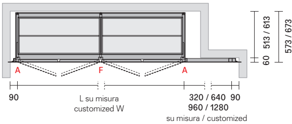
composizione lineare con contenitore laterale linear composition with side storage unit
