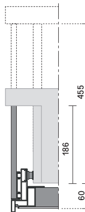
passaggio completo E45 complete passage E45 estensibile da mm 186 a mm 455 extensible from mm 186 to mm 455
