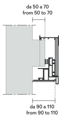
fascia terminale con fascia di aggiustaggio laterale terminal closing filler with adjustable lateral filler
