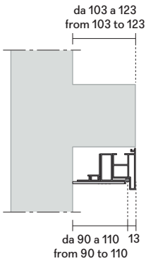
profilo terminale con fascia di aggiustaggio laterale terminal profile with adjustable lateral filler
