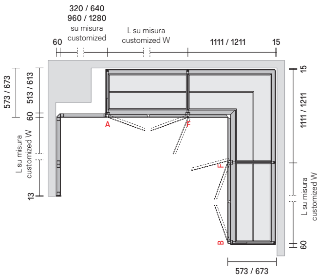
composizione articolata con contenitore angolare articulated composition with corner storage unit
