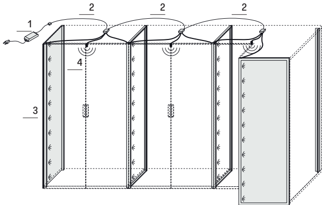
illuminazione anteriore / front led lighting
