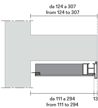
profilo terminale con fascia laterale su misura terminal profile with customized lateral filler
