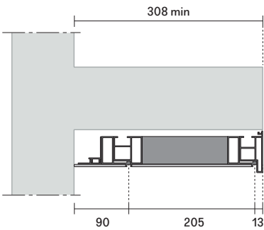
profilo terminale con fascia di aggiustaggio laterale e pannello / terminal profile with adjustable lateral filler and panel
