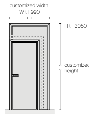
Swing door
